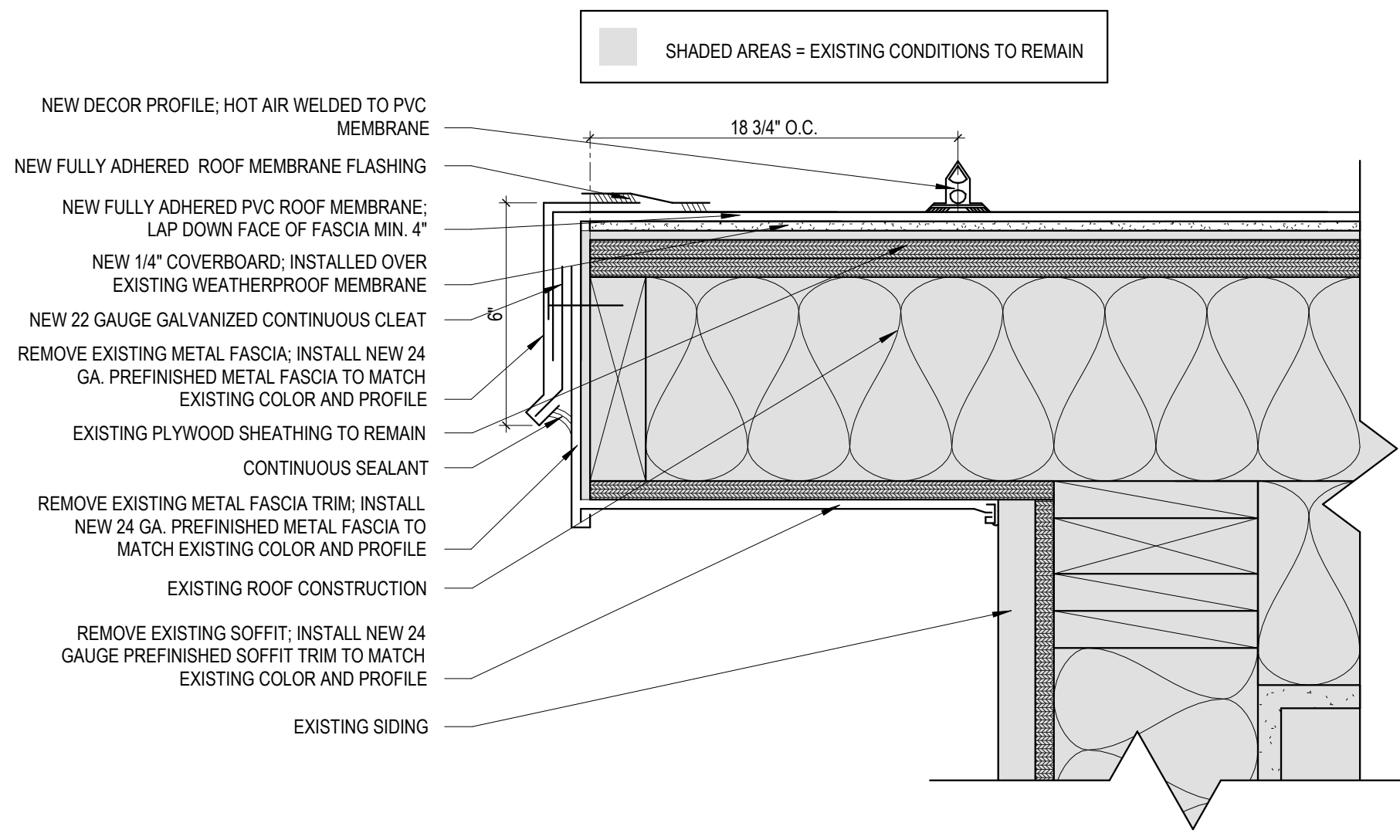
5 Fascia Detail Scale: 3" = 1'-0"
