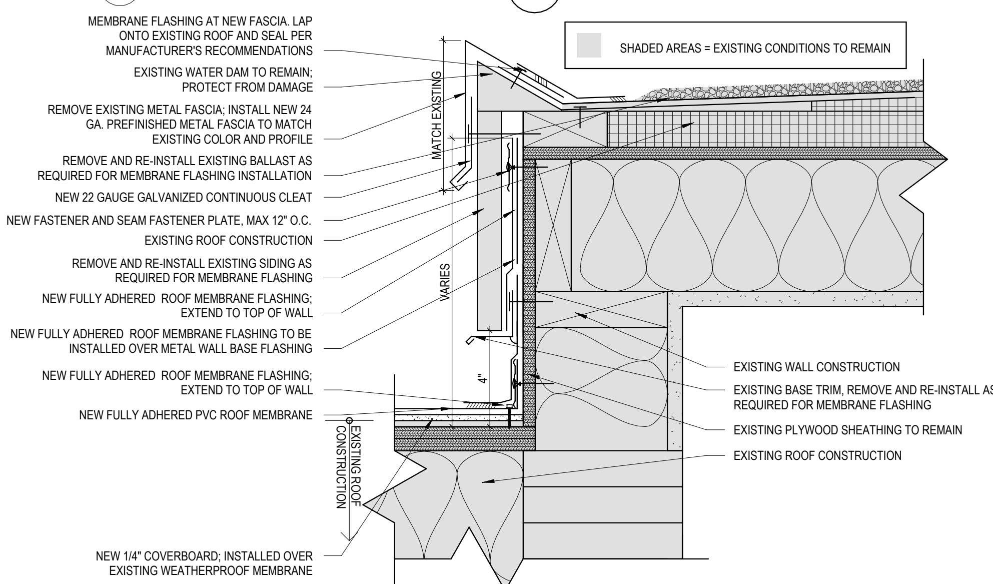
4 Fascia Detail Scale: 3" = 1'-0"
