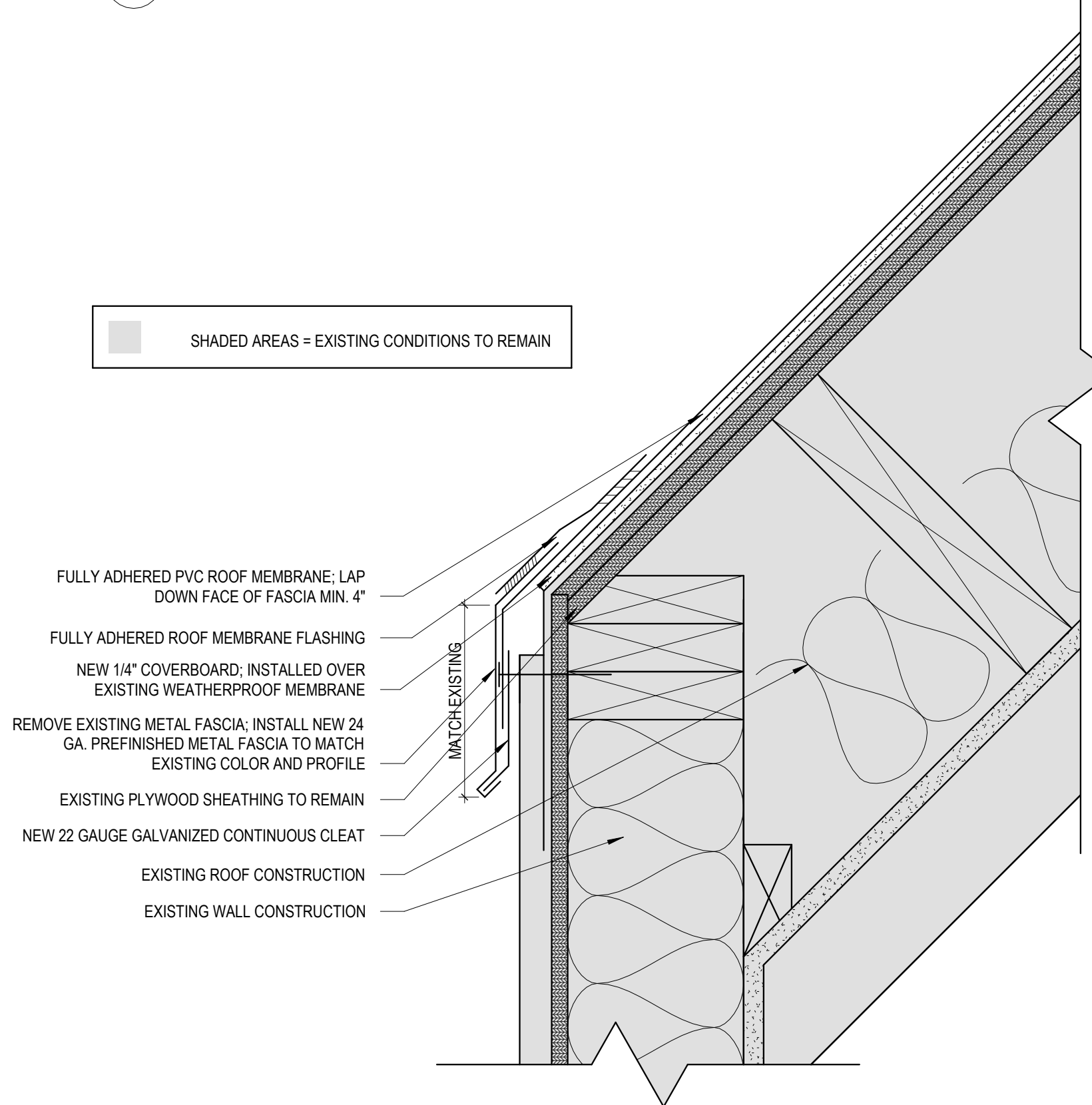
3 Fascia Detail Scale: 3" = 1'-0"
