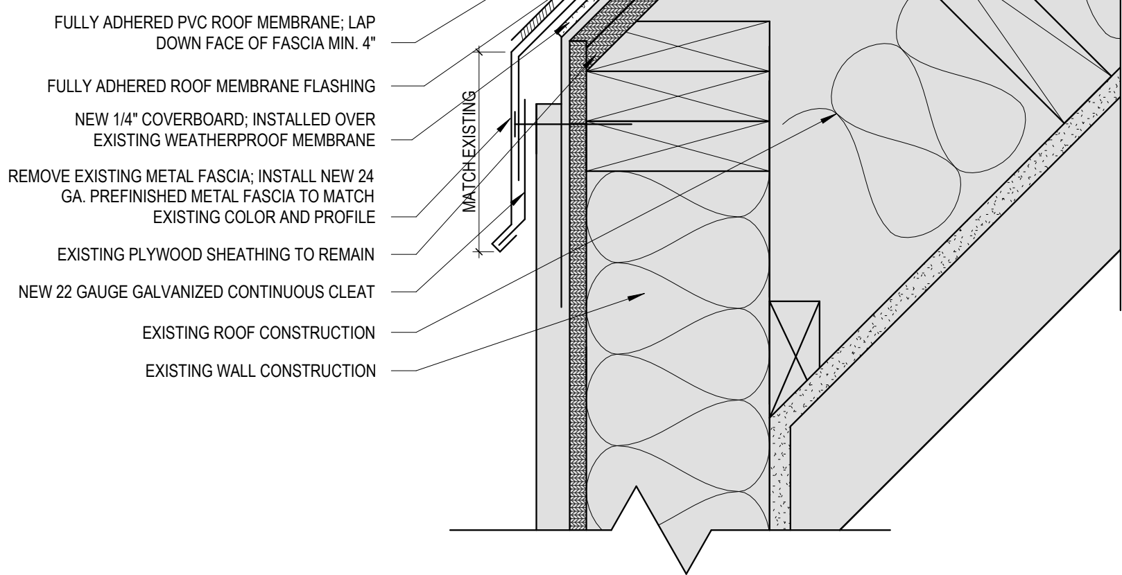
3 Fascia Detail Scale: 3" = 1'-0"
