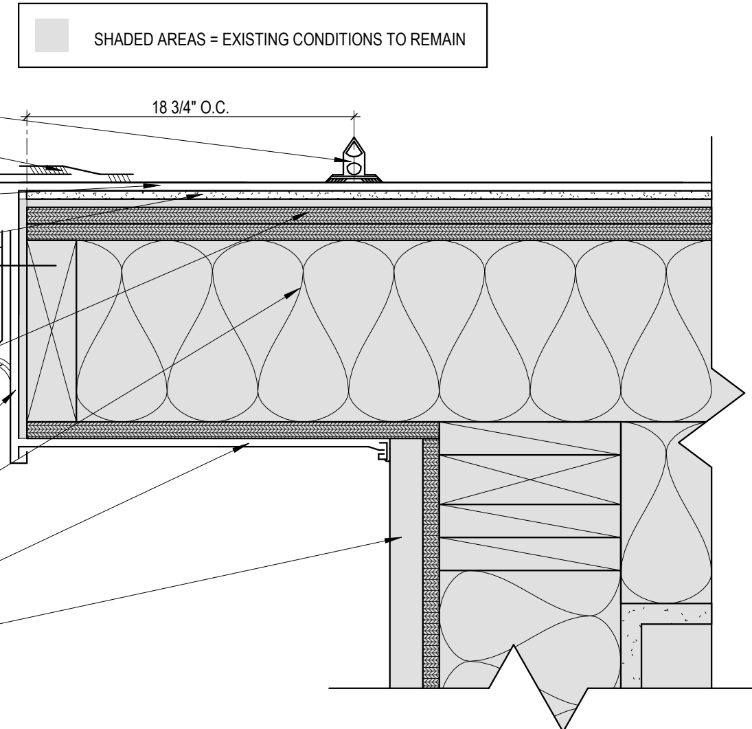
5 Fascia Detail Scale: 3" = 1'-0"
